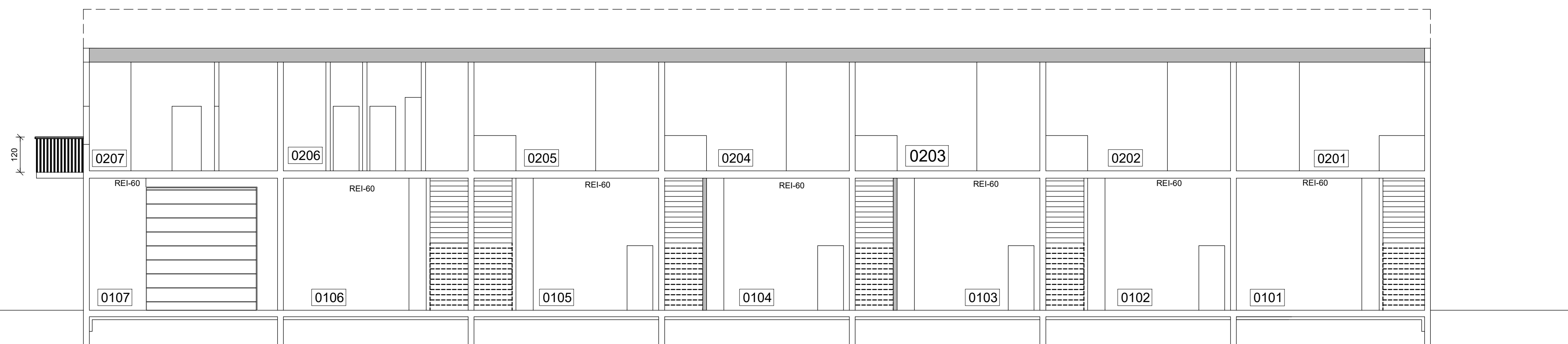
Sniď C-C 1/100
