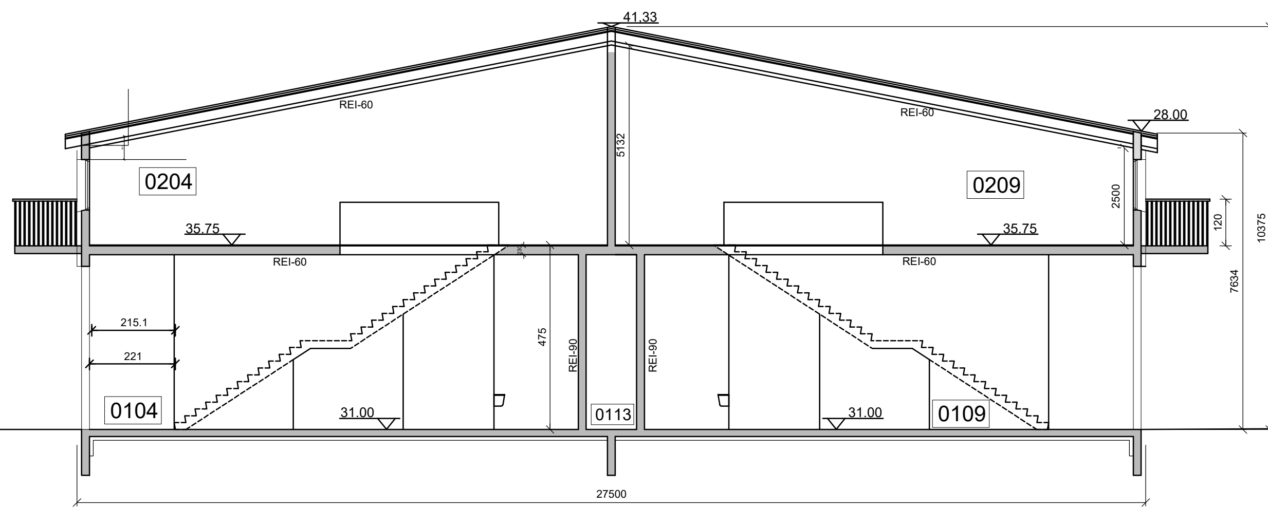
Sniž A-A 1/100
