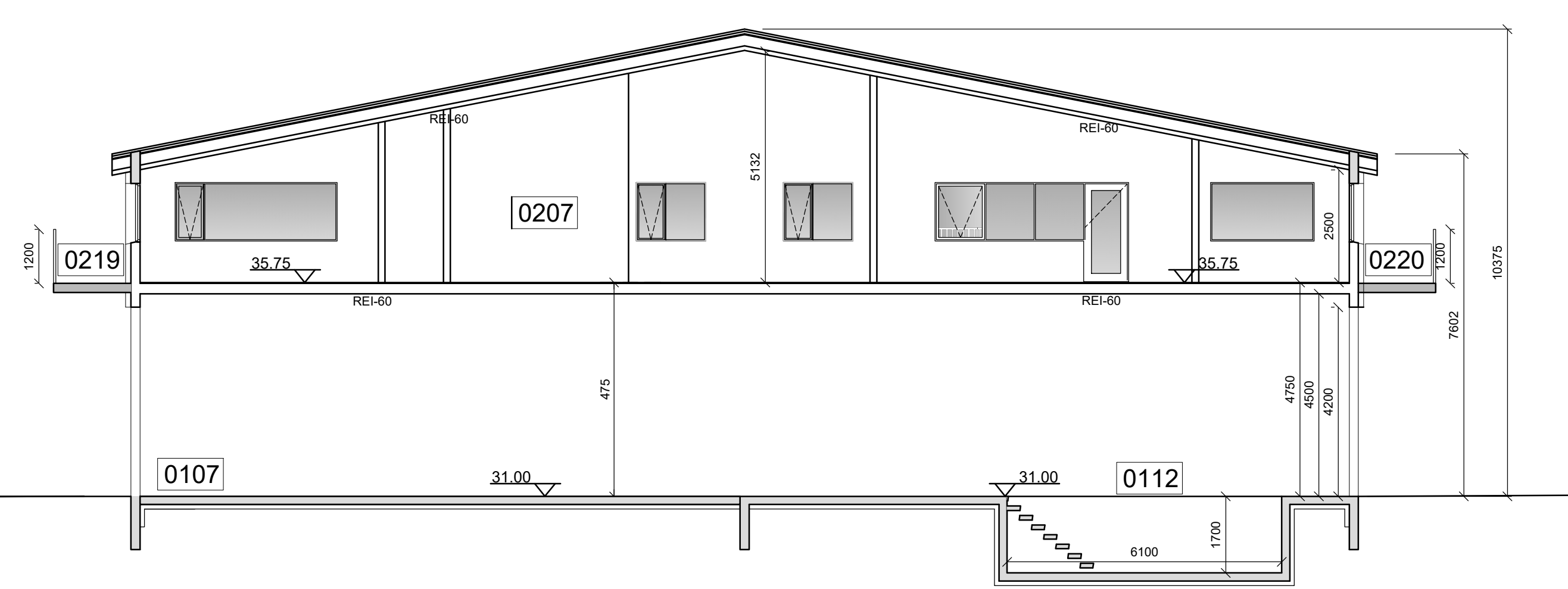
Sniž B-B 1/100
