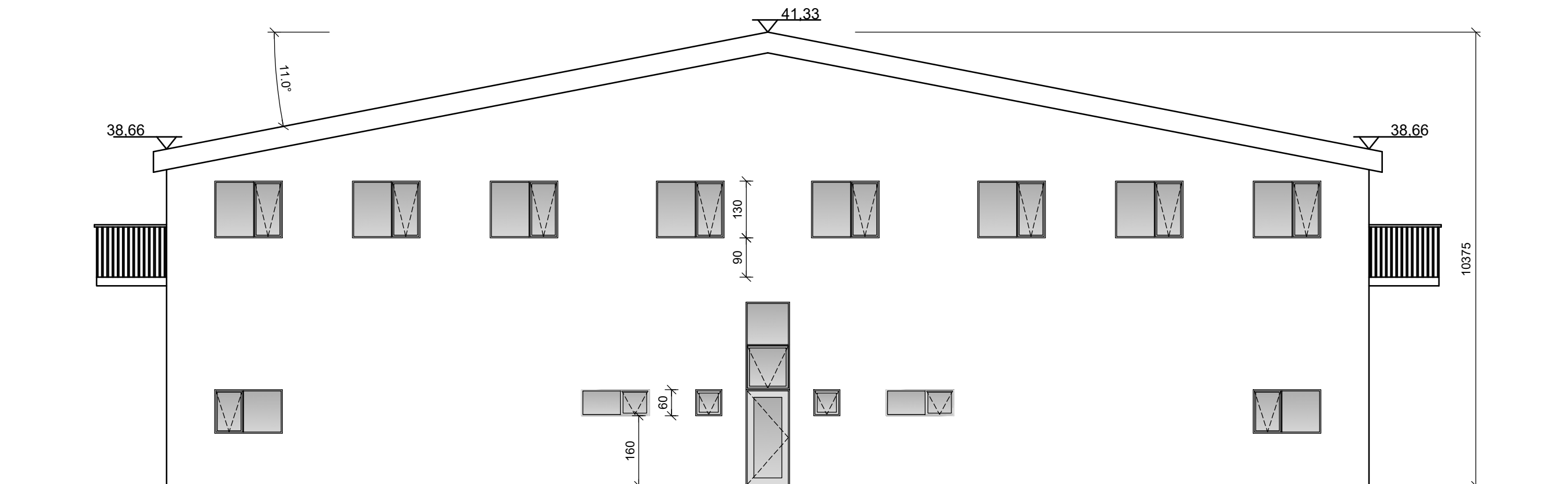
Útlit suður 1/100
