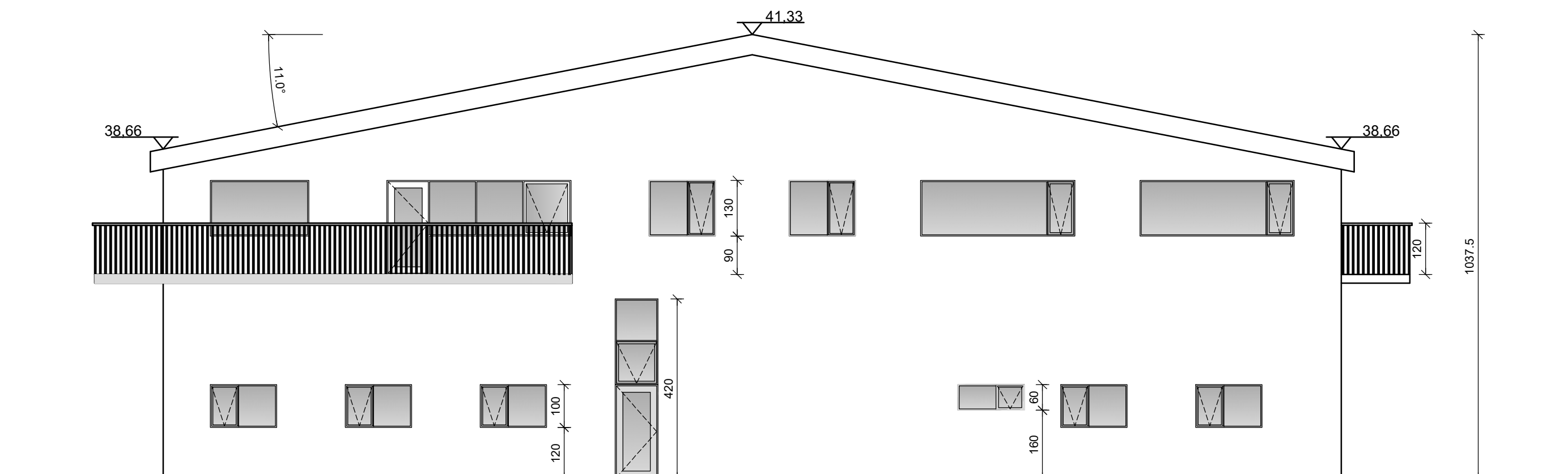
Útlit norður 1/100
